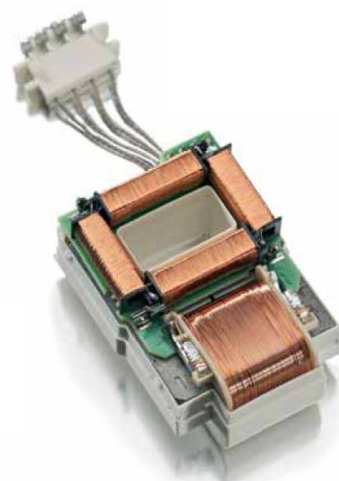
Встроенные трансформаторы тока
