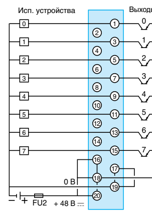
FU2: быстродействующий плавкий предохранитель 10 А
