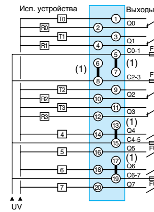
UV: 19...240 В ~ или 19...60 В --- для TSX DSY 08R5A, 24...130 В --- для TSX DSY 08R4D FU: быстродействующий плавкий предохранитель 6,3 А (1) Подключение должно осуществляться для питания 24 В --- или 24 В ~
