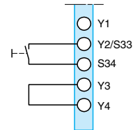
Ручной сброс без контроля пусковой кнопки
