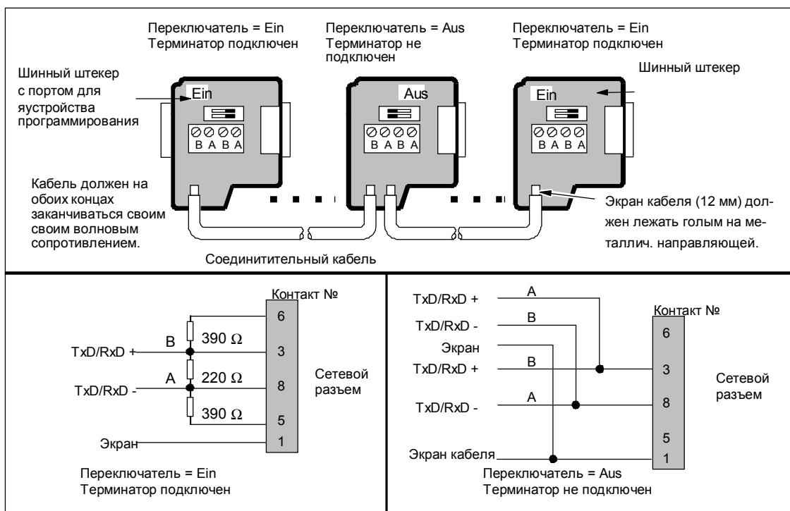
Рис. 8-3. Соединительный кабель с ТЕРМИНАТОРОМ
