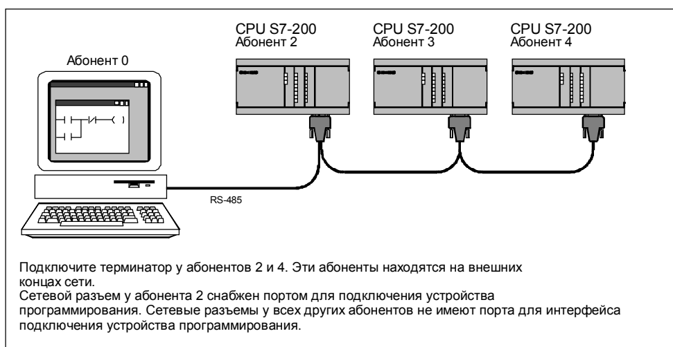
Рис. 8-5. Обмен сообщениями в сети через PC с платой MPI
