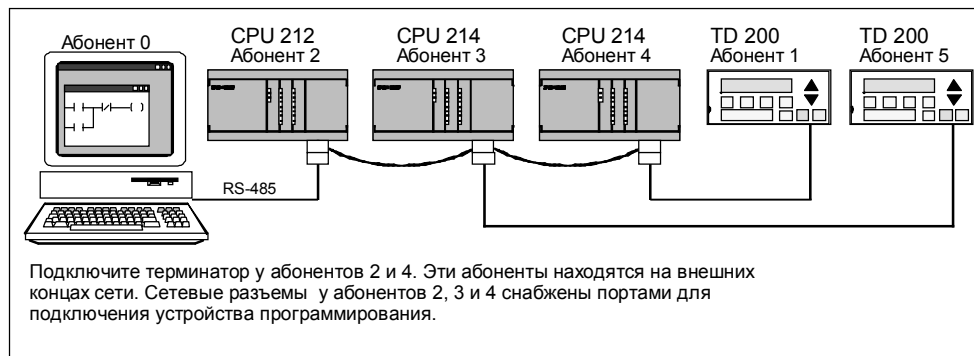
Рис. 8-6. Два дополнительных текстовых дисплея TD 200 в сети
