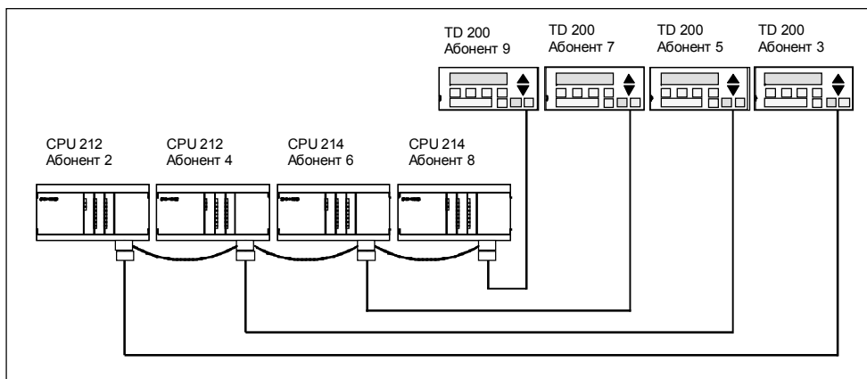
Рис. 8-7. Пример сети с передачей маркера
