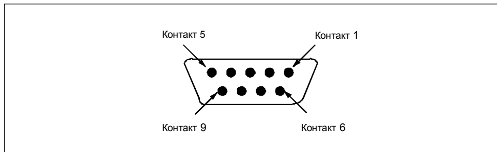
Рис. 8-1. Штекер коммуникационного порта S7-200
