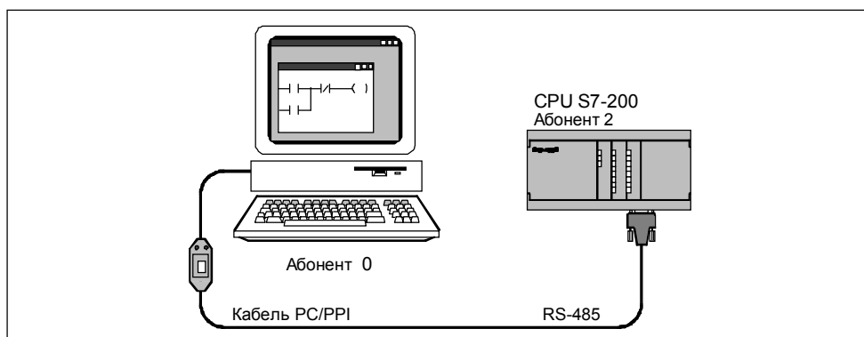
Рис. 8-2. Обмен сообщениями с CPU S7-200 через кабель PC/PPI
