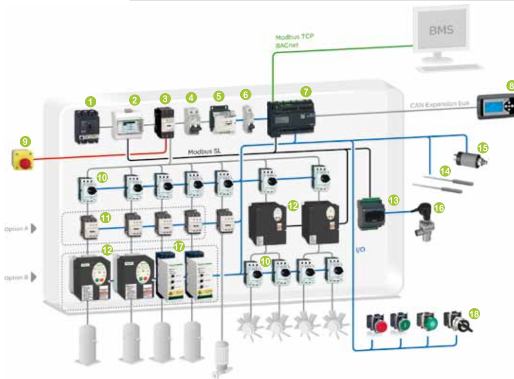
Управление компрессором
