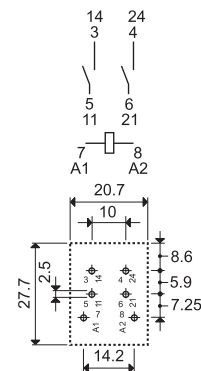
56.42-0300 Вид сбоку
