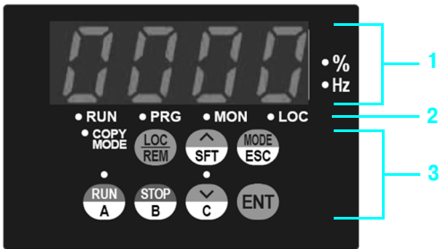
Передняя панель выносного терминала
