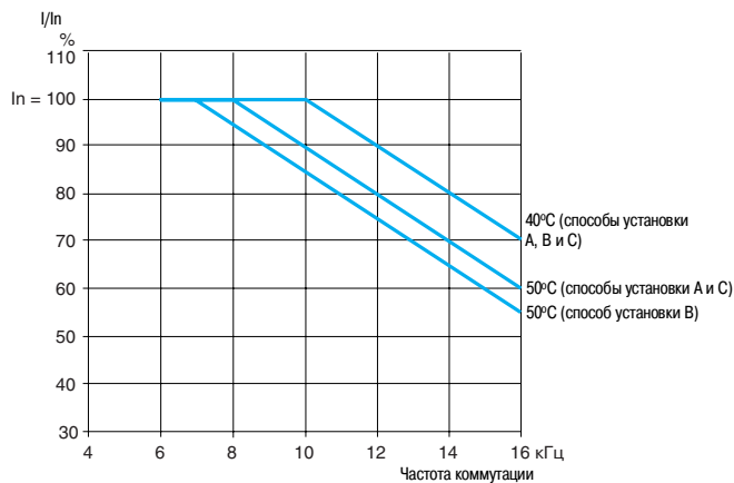
ATV 21HD22N4
