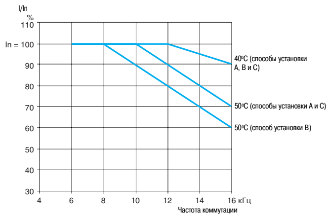
ATV 21HD18N4
