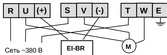
Модель EI-P7012-200H...EI-P7012-450H (160...370 кВт)
