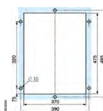
Частично утопленный монтаж
