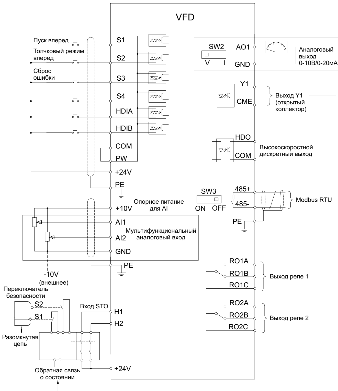
Рис 4.15 Схема подключения цепей управления
