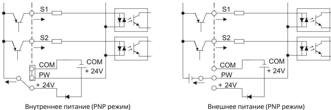
Рис 4.18 PNP режим
