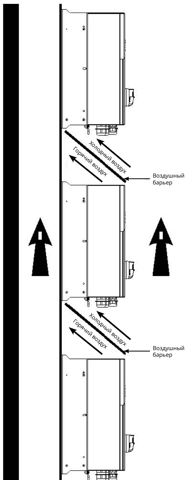
Рис 4.5 Вертикальная установка
