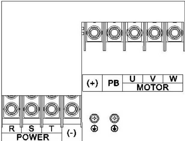
Рис 4.13 75-110 кВт
