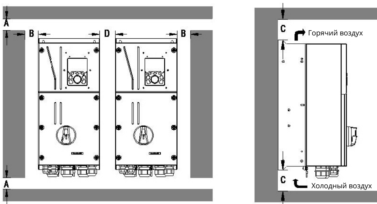
Рис 4.4 Параллельная установка
