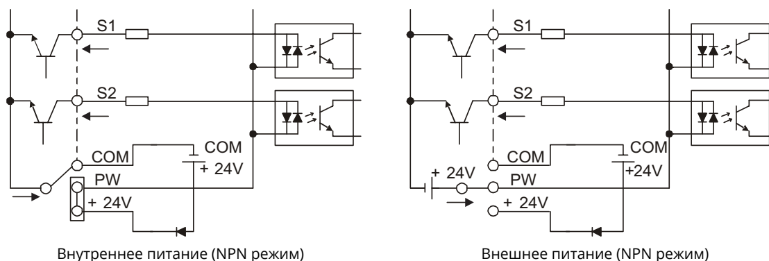
Рис 4.17 NPN режим
