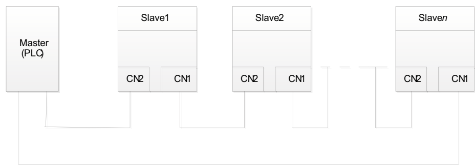
Рисунок А.10 Электрическая схема подключения кольцевой сети
