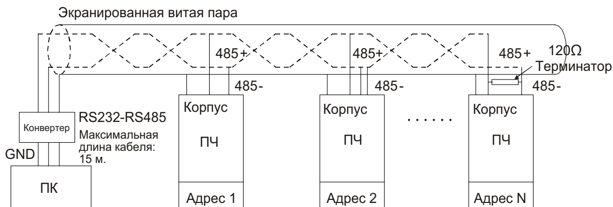
Рис 9.4 Практическая схема
