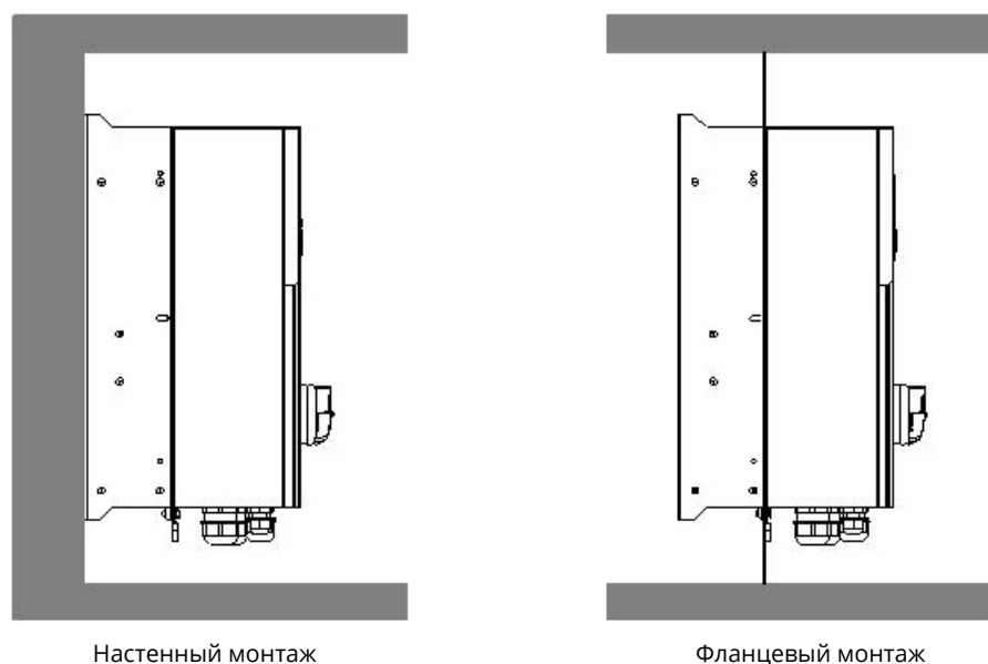
Рис 4.2 Способы установки
