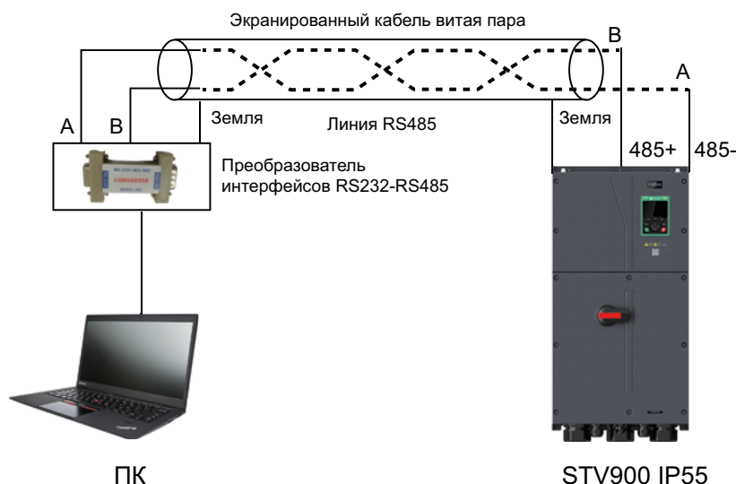
Рис 9.1 Подключение RS485 к одному ПЧ
