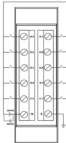
Дискретные входы контроллера SM253CE10
