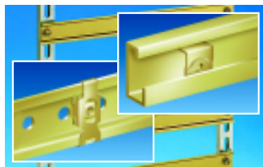
Шасси в сборе со стойками и боковыми перекладинами
