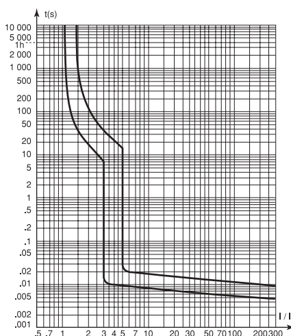
NG125, кривая В
