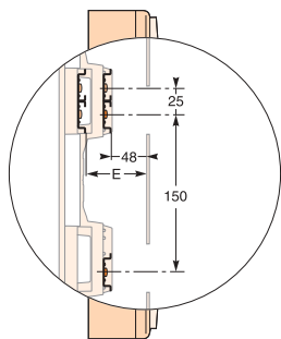
Два варианта установки DIN-рейки по глубине
