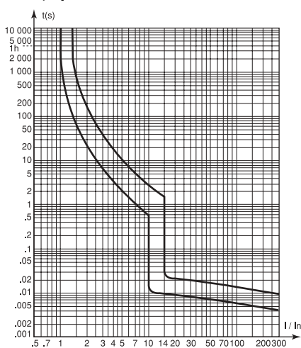
С60, кривая D
