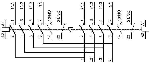
Электрическая блокировка реверсивных контакторов, оснащенных: механической блокировкой со встроенными электрическими контактами LA9-D●●●02
