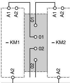
Комплект соединения контакторов управления 2-х скоростными двигателями
