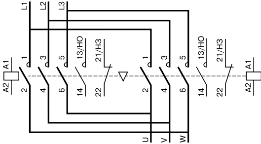
Реверсивные контакторы для управления двигателями, горизонтального крепления LC2-D09...D150
