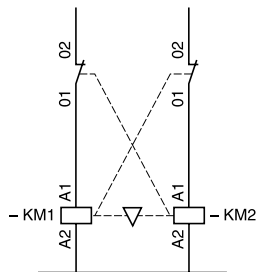
Комплект соединения контакторов управления 2-х скоростными двигателями
