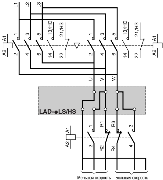
Комплект соединения контакторов управления 2-х скоростными двигателями
